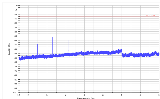
LTE Band 5 10MHz CH-Middle 1.5GHz~9GHz
