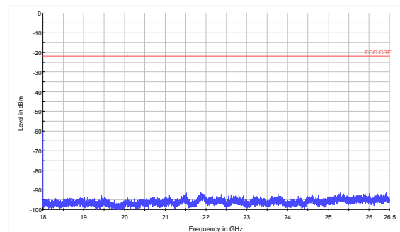
GFSK-CH78 18GHz to 26.5GHz
