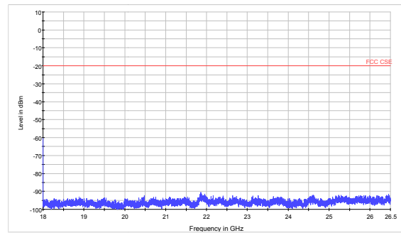
EDR-CH78 18GHz to 26.5GHz
