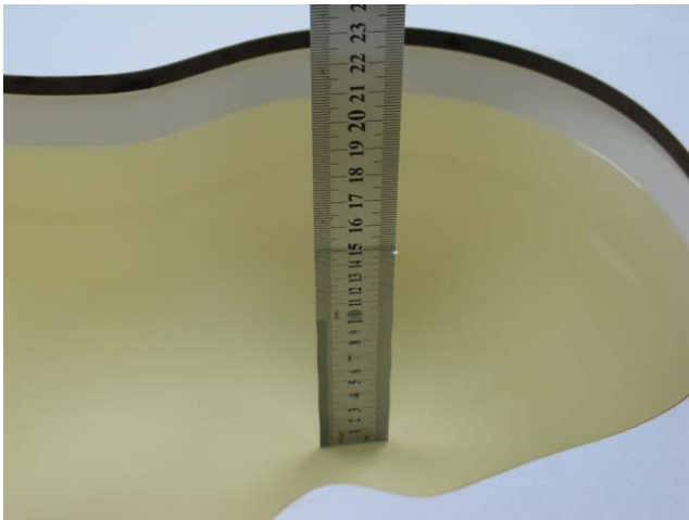
Photo 19: HSL2450MHz depth (15cm)
