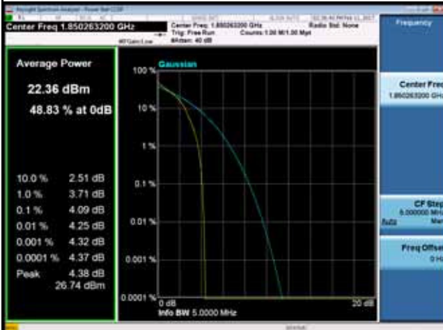
QPSK-19193
