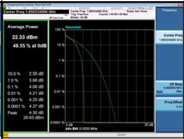
16QAM-19185
