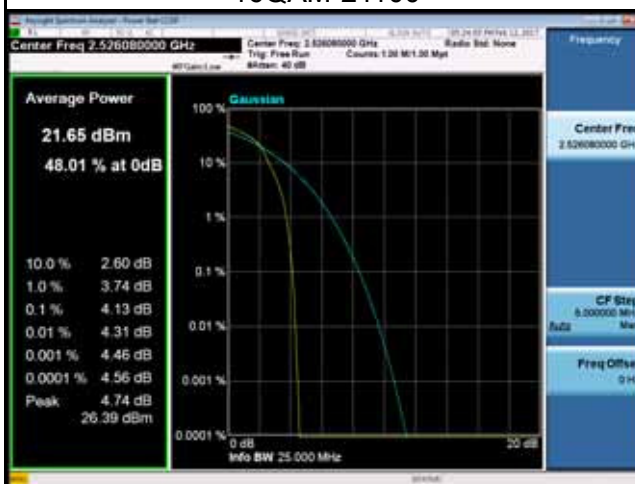
16QAM-21100
