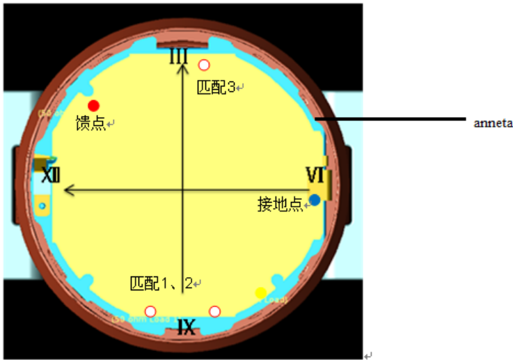
图（b）天线馈电点示意图
