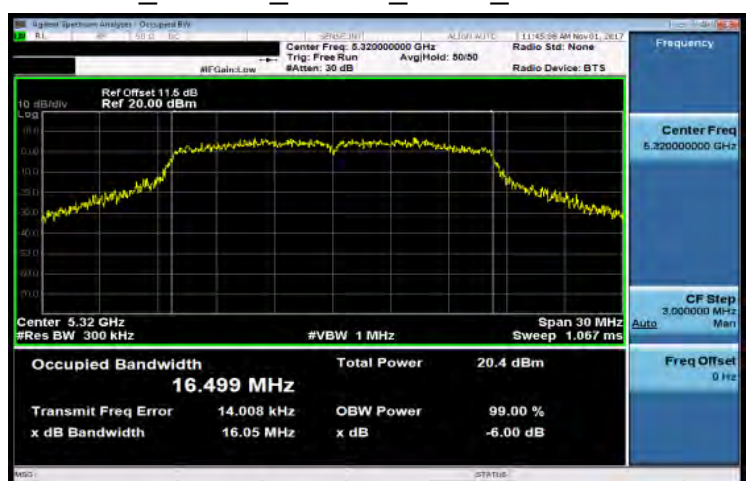
IC_802.11a_20MHz_AUX1_5320MHz
