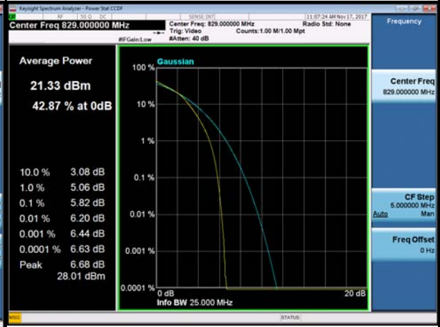
16QAM-26990
