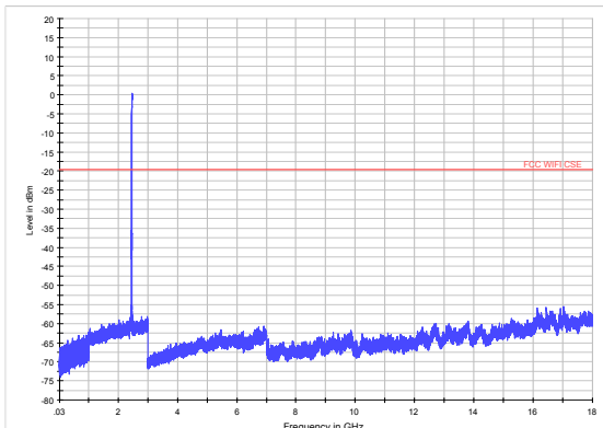
802.11b CH10 30MHz to 18GHz
