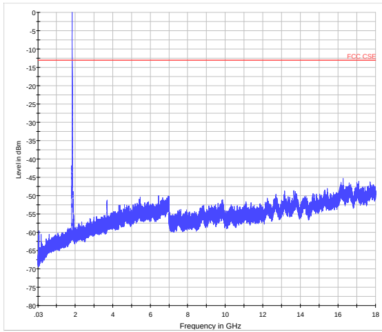
WCDMA Band II CH-Middle 30MHz~18GHz
