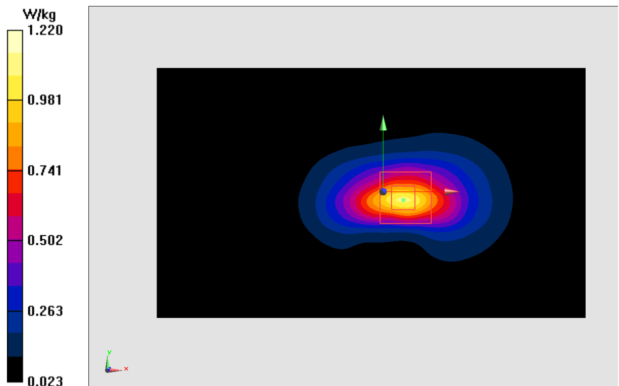
Fig.14 LTE Band4
