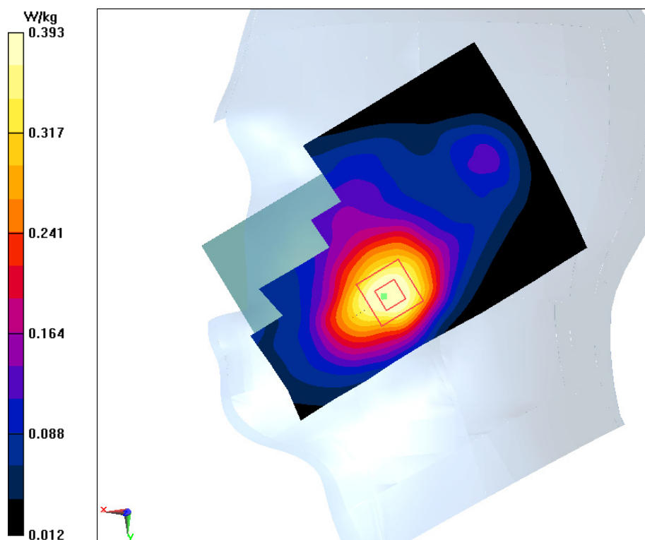
Fig.7 1700MHz
