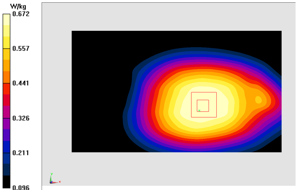
Fig.6 WCDMA 850
