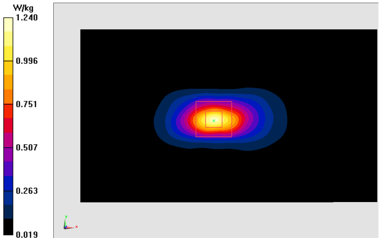
Fig.12 LTE Band2
