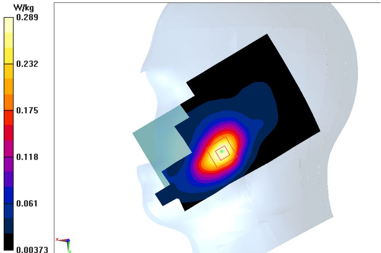
Fig.9 WCDMA1900
