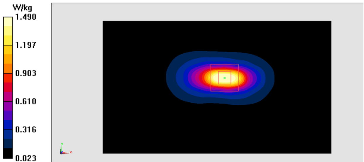
Fig.10 WCDMA1900
