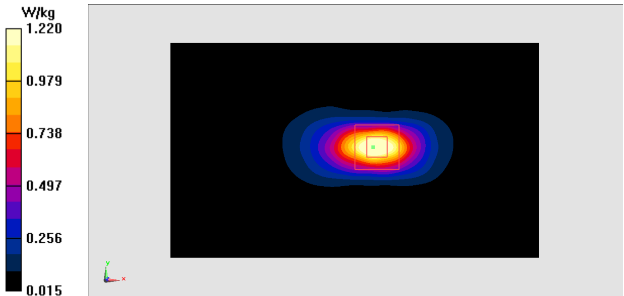
Fig.12 LTE Band2
