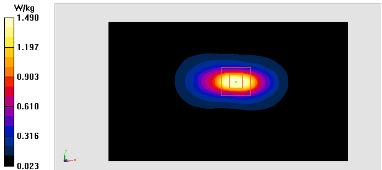
Fig.10 WCDMA1900
