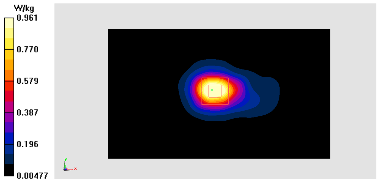
Fig.18 LTE Band7
