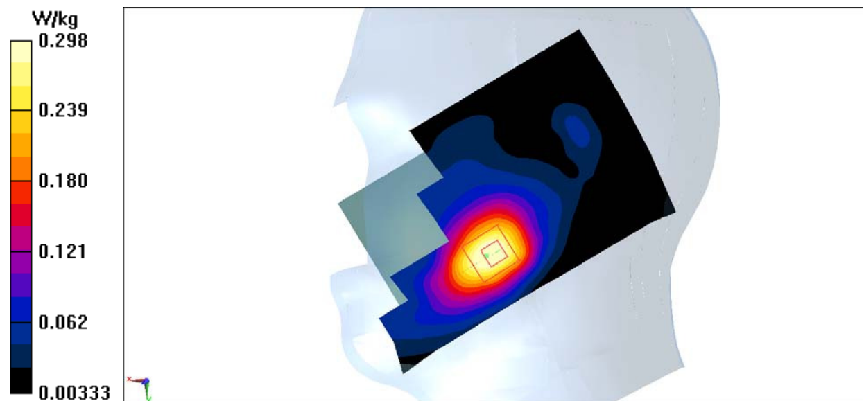
Fig.9 WCDMA1900
