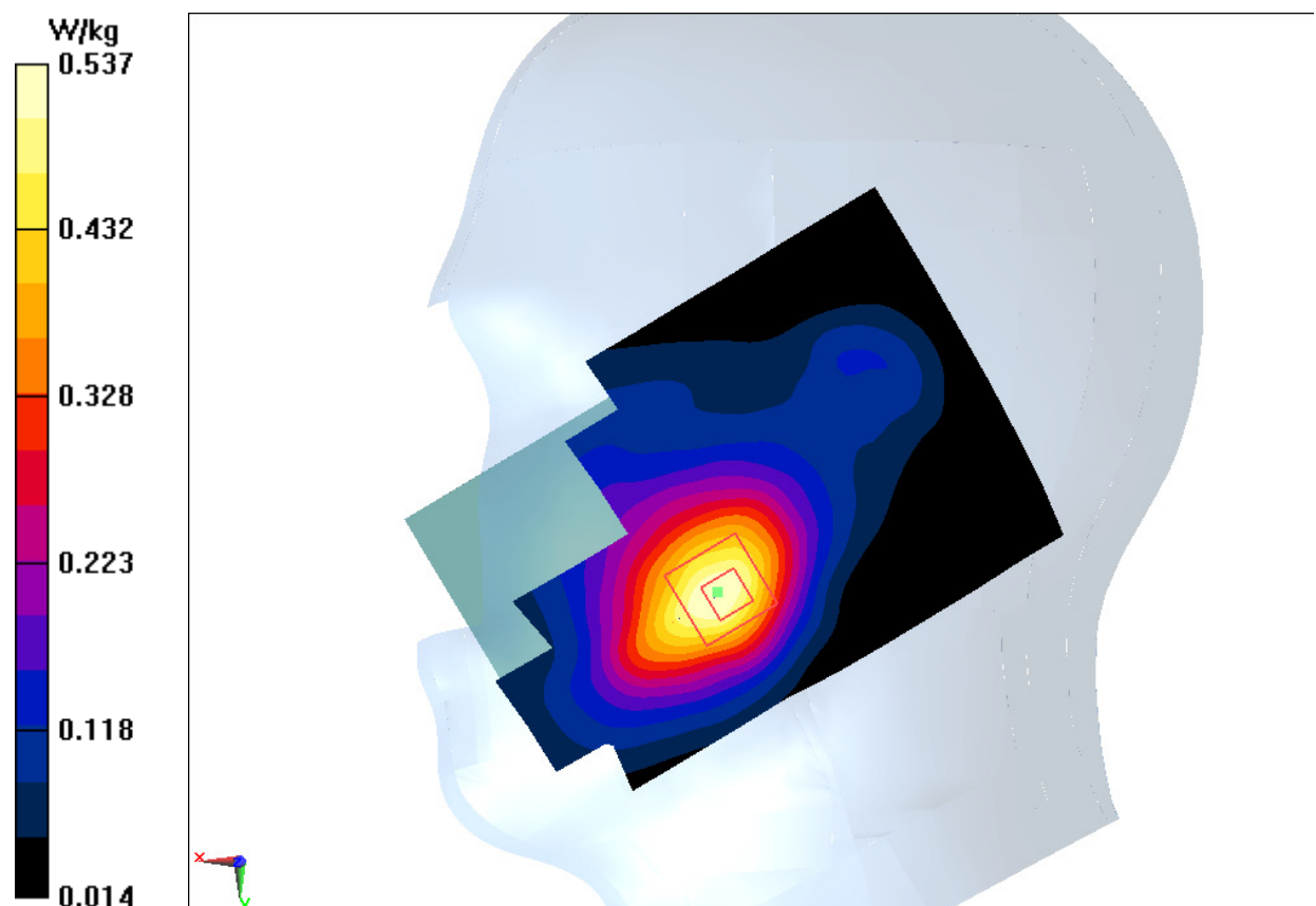
Fig.7 1700MHz
