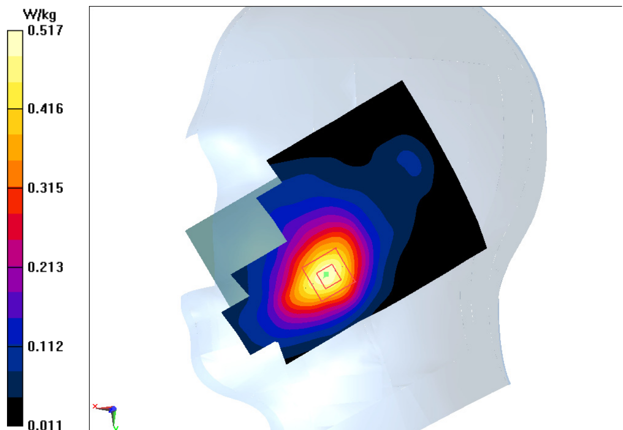
Fig.13 LTE Band4
