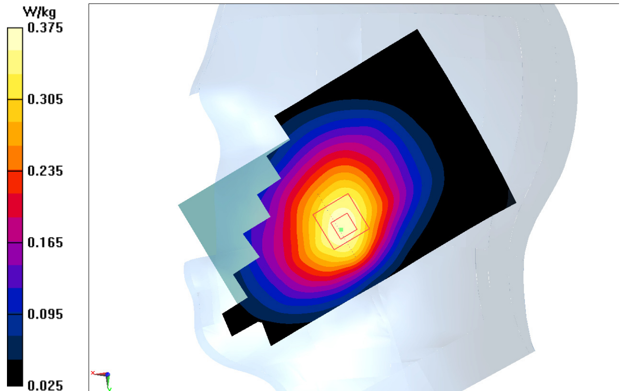
Fig.5 WCDMA 850
