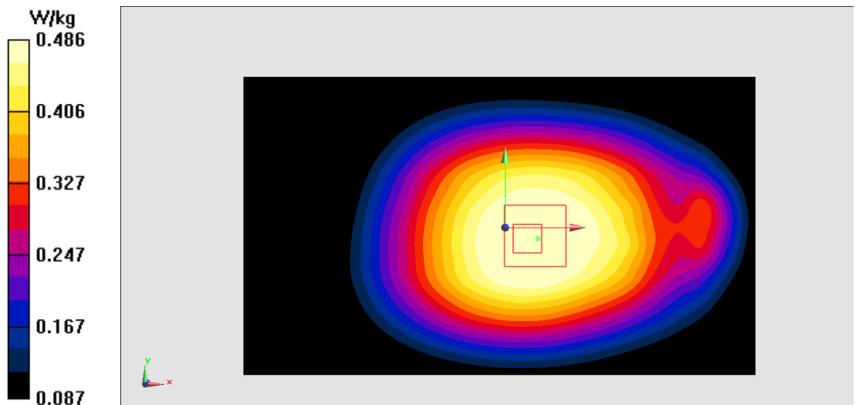
Fig.16 LTE Band5
