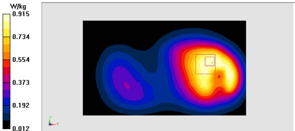
Fig.14 LTE Band4
