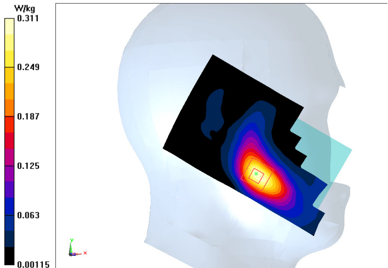
Fig.17 LTE Band7
