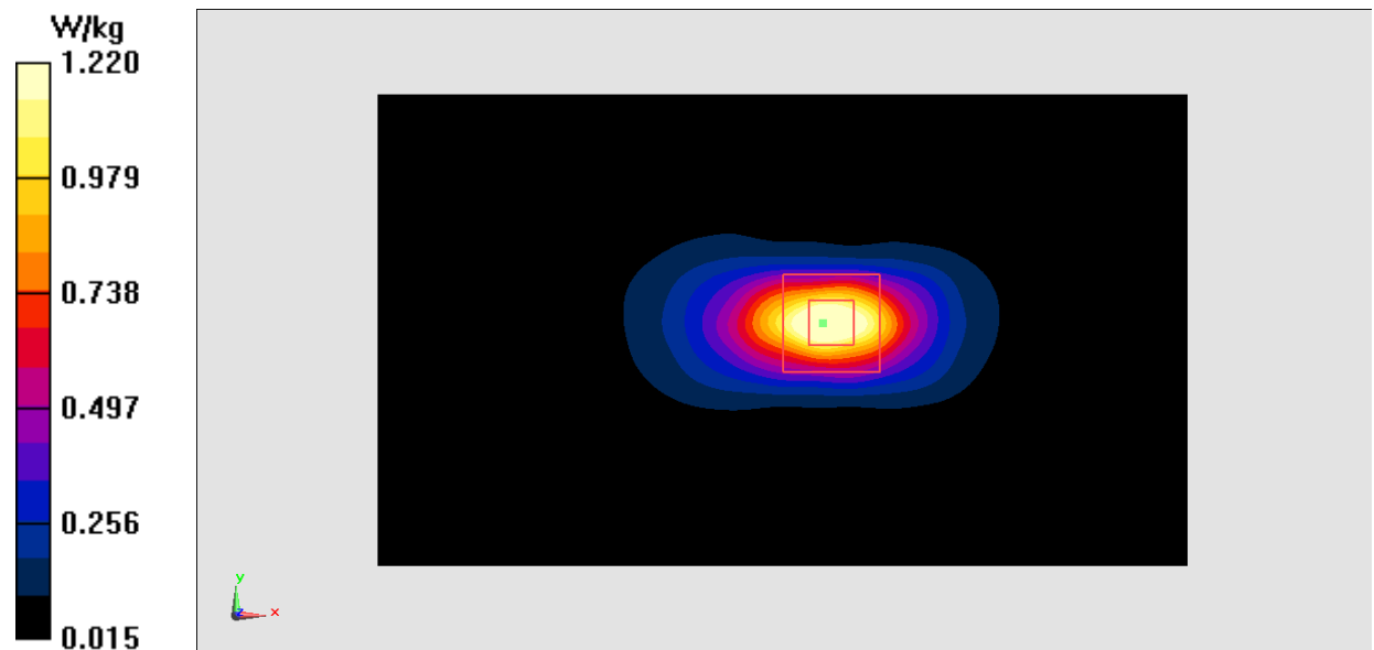
Fig.12 LTE Band2
