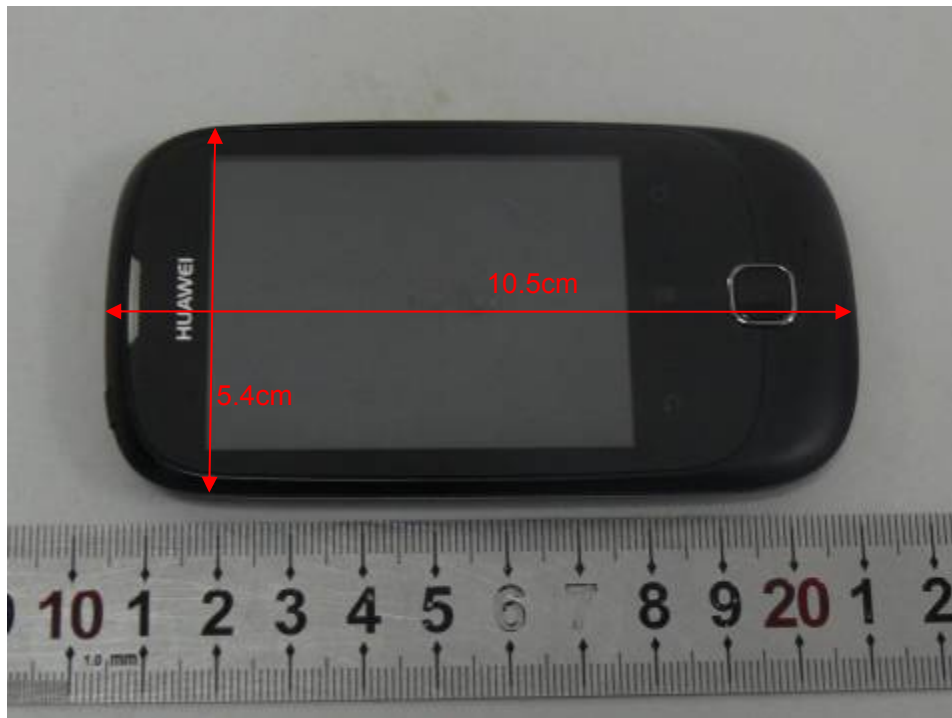
a: EUT
