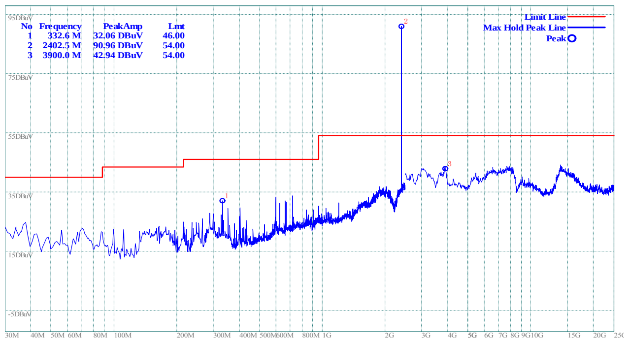
(Plot A.1: Antenna Horizontal)
