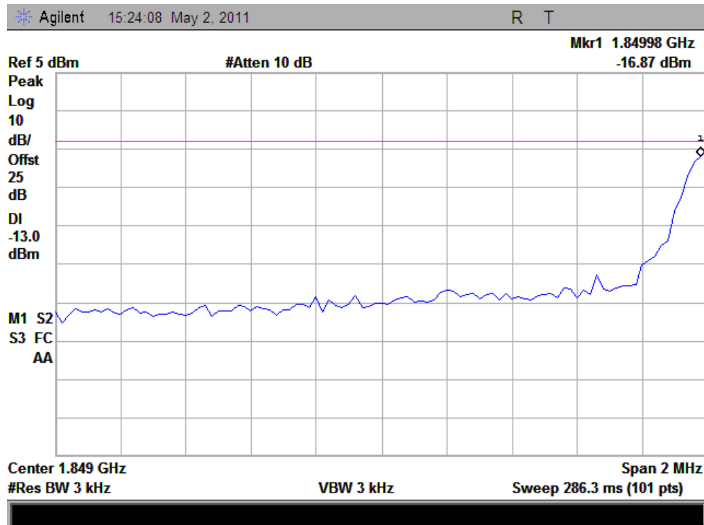
(Plot A: GSM1900, Channel = 512)
