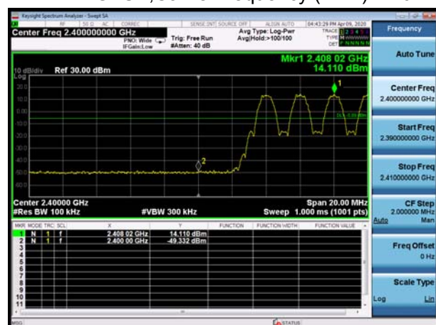
BLE 2M GFSK,Carrier frequency (MHz): 2404
