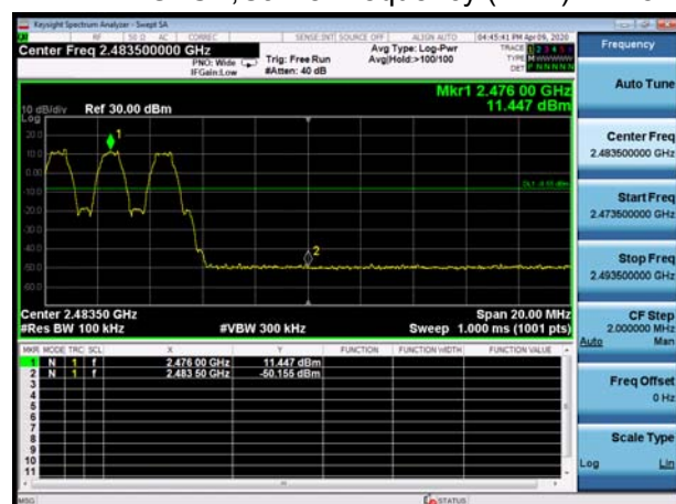
BLE 2M GFSK,Carrier frequency (MHz): 2478
