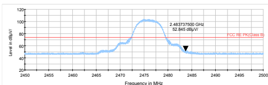
BT UHD 4M \pi/4 -DQPSK 2476MHz: Peak
