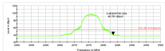
BT UHD 4M \pi/4 -DQPSK 2476MHz: Average
