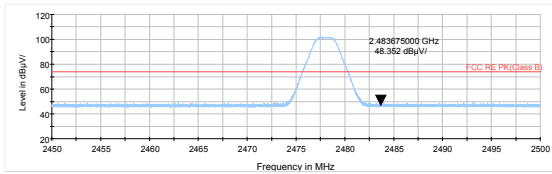
BLE 2M GFSK 2478MHz: Peak
