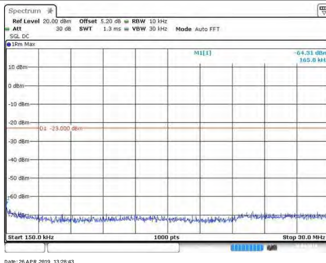
GSM850_190
