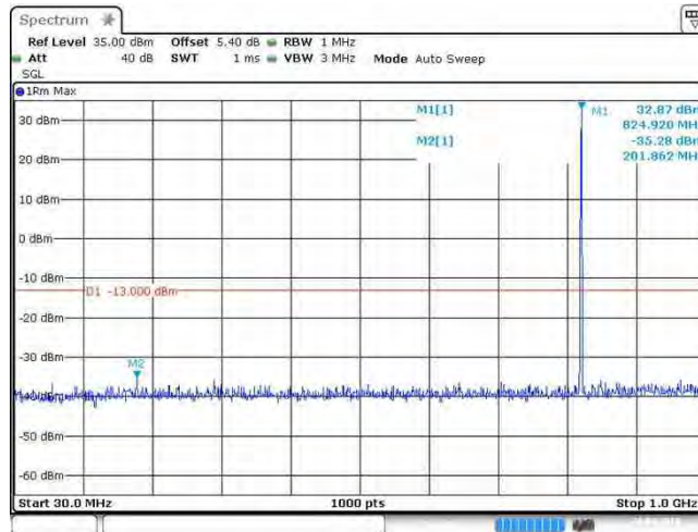
GSM850_128
