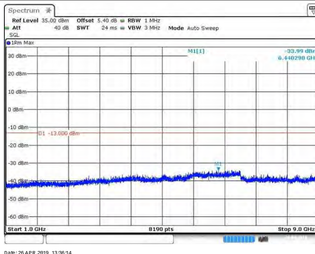
EGPRS850_190
