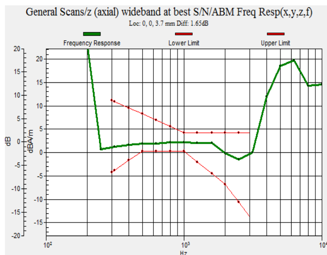
UMTS Band II/9400CH(battery 1#)
