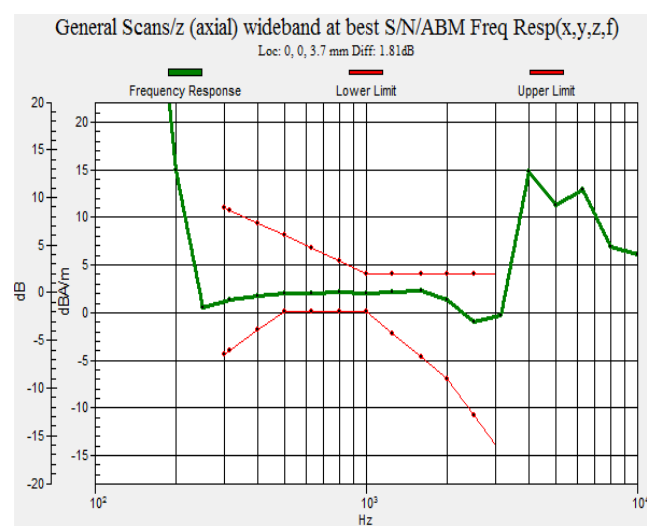
UMTS Band II/9400CH(battery 2#)
