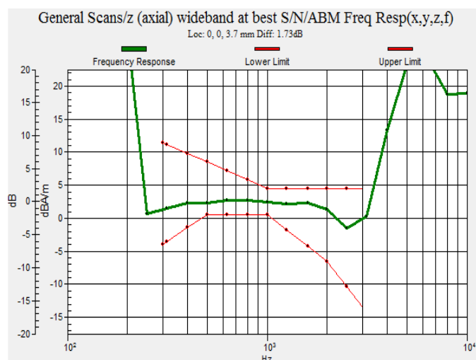
GSM1900/661CH(battery 1#)
