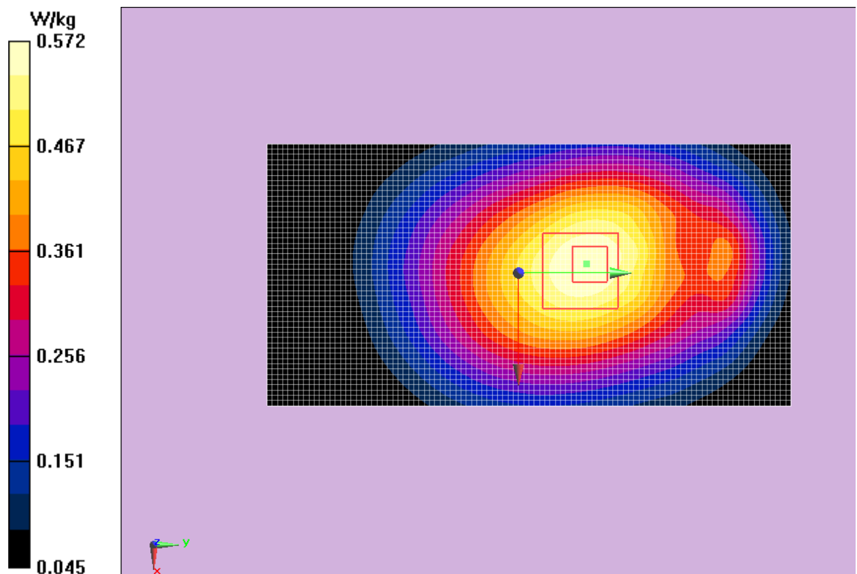
Fig.6 WCDMA 850
