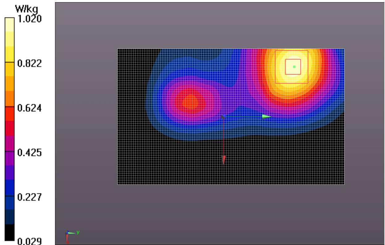
Fig.8 WCDMA1900 CH9262
