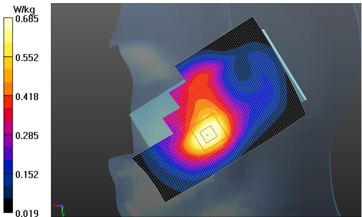
Fig.7 WCDMA1900 CH9400
