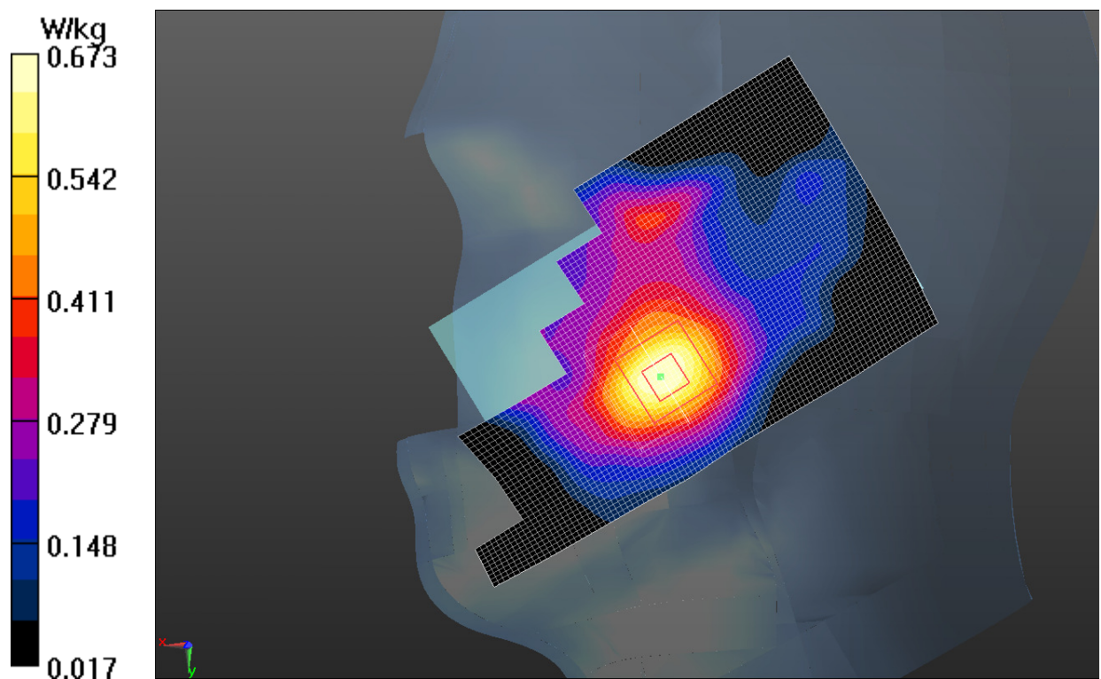
Fig.7 WCDMA1900 CH9400
