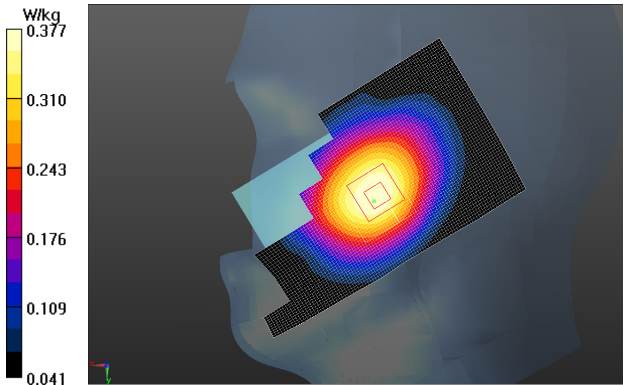
Fig.5 WCDMA 850 CH4183
