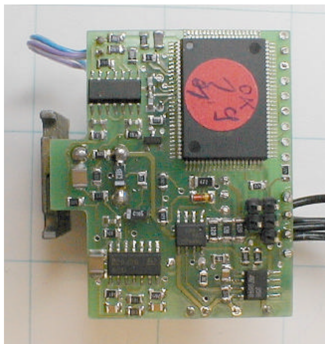
PCB Bottom
