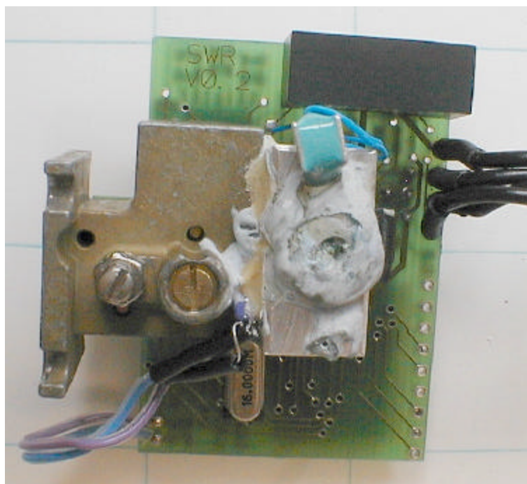
PCB Top
