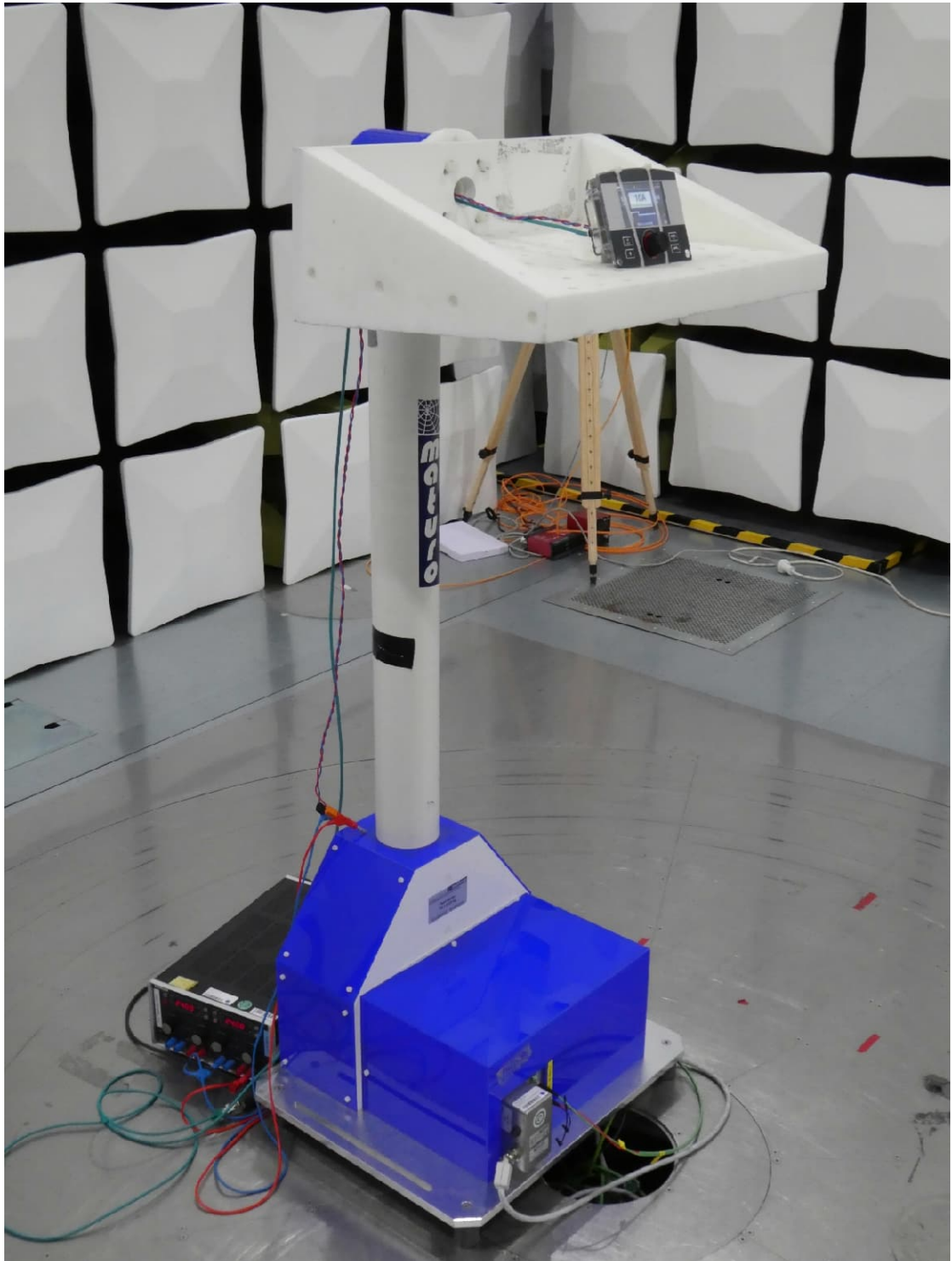
EUT setup – f > 1 \text{ GHz}
