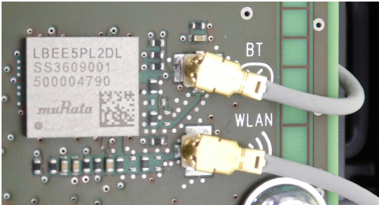
Radio module
