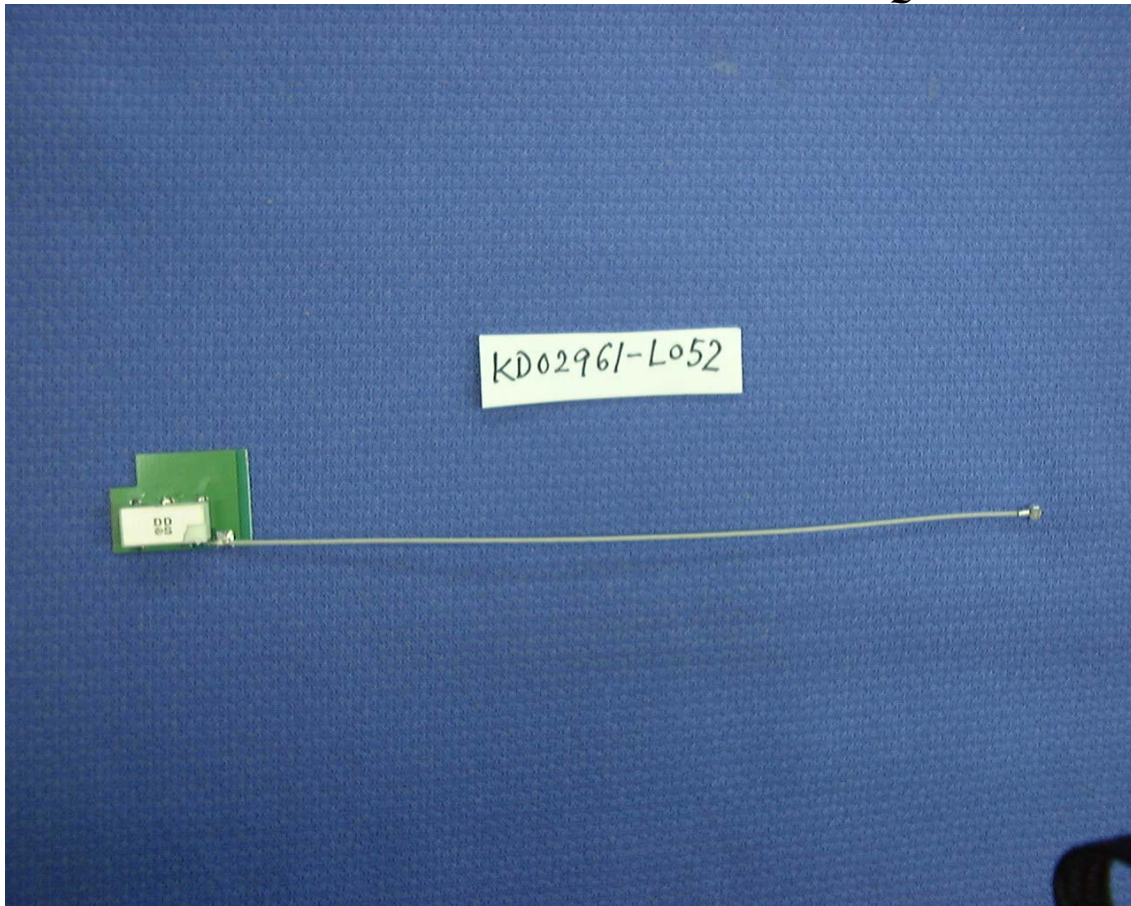
Antenna (KD02961-L052)
