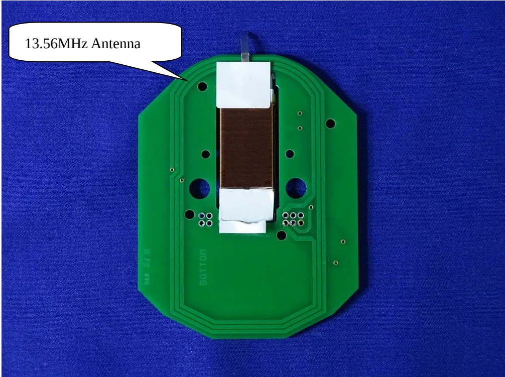
(15) EUT Photo
