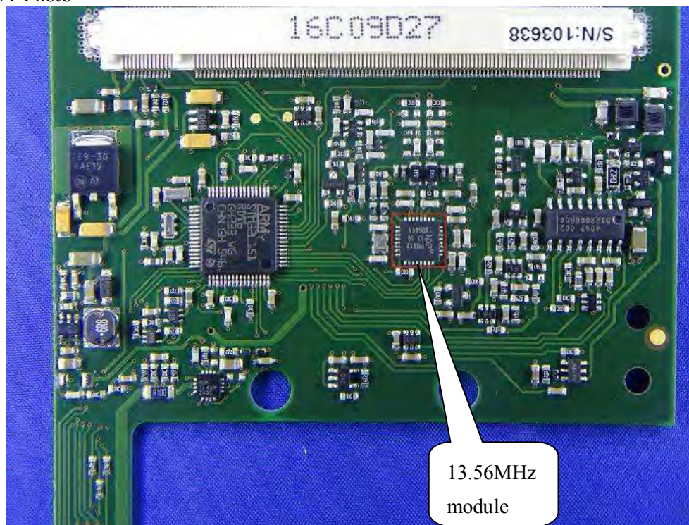
(16) EUT Photo
