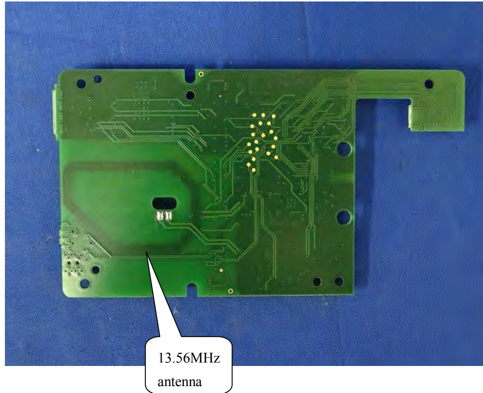
(20) EUT Photo
