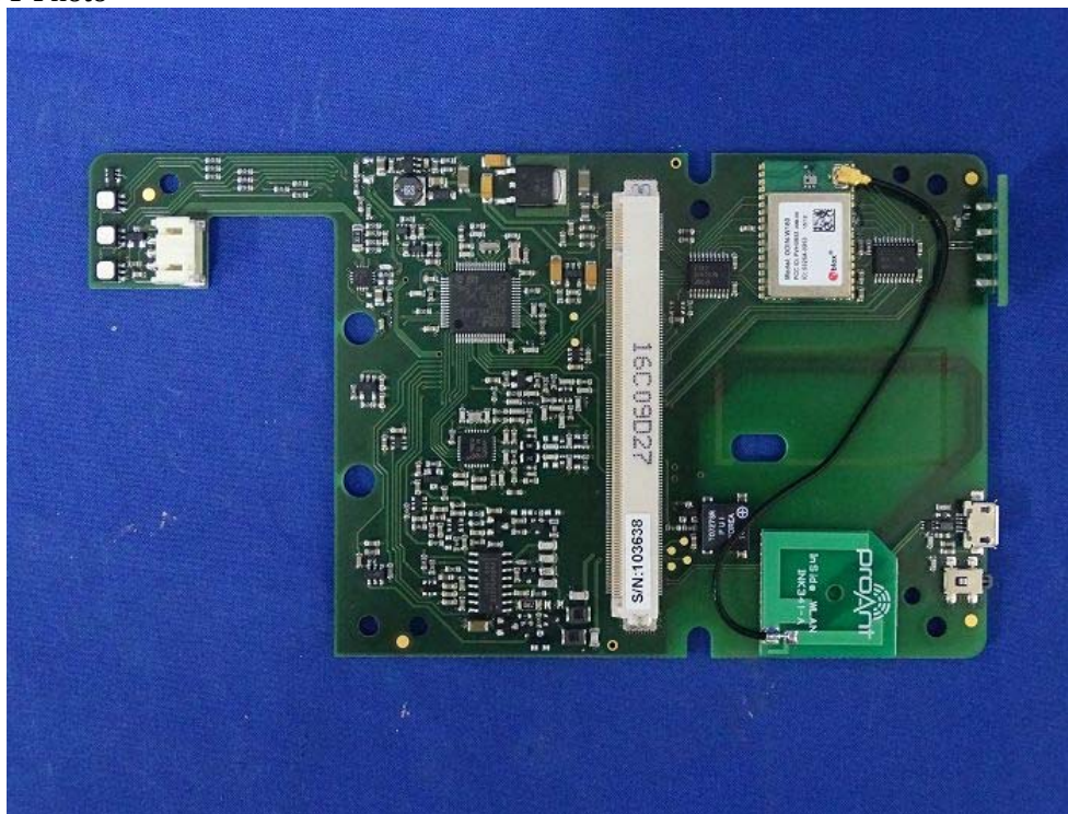
(13) EUT Photo
