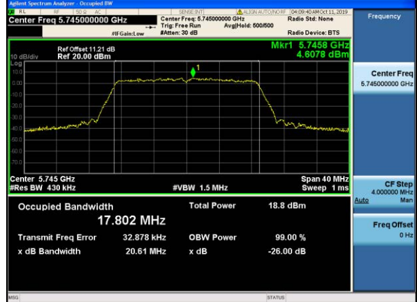
11n(HT20) CH149
