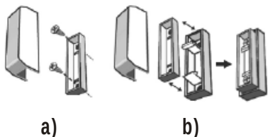
Fig. 2 – Installazione del magnete: a) SENZA distanziatore; b) CON distanziatore. Magnet installation: a) with NO spacer; b) WITH spacer Installation de l'aimant: a) SANS espace-leur; b) AVEC espace-leur.
