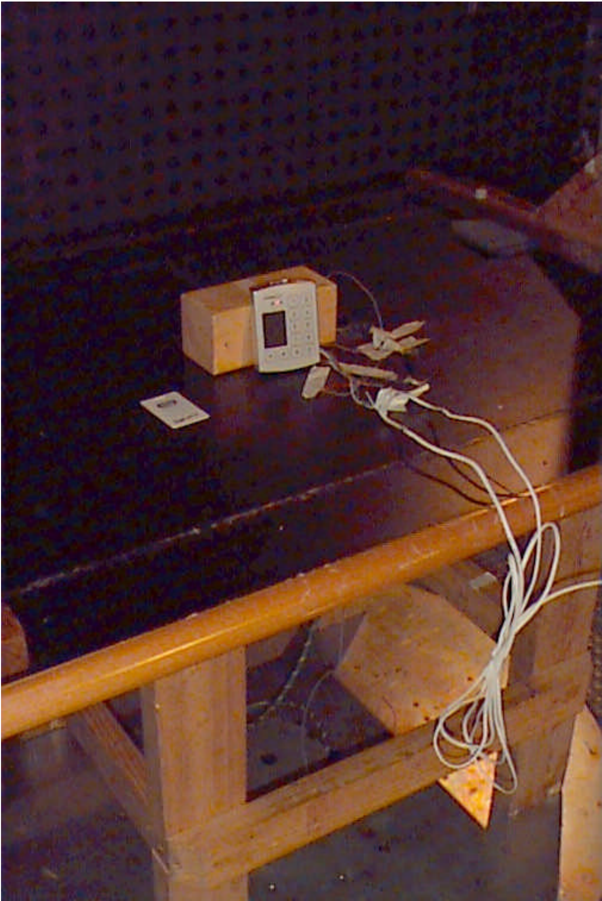
EUT test configuration
