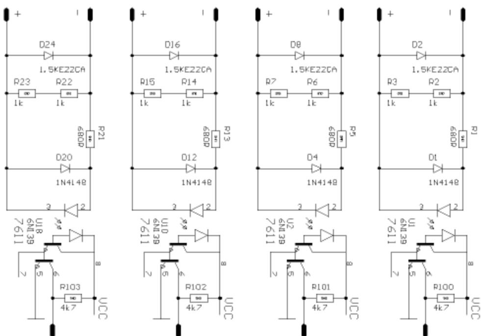
TTL-Seite/serielle Schnittstellen
