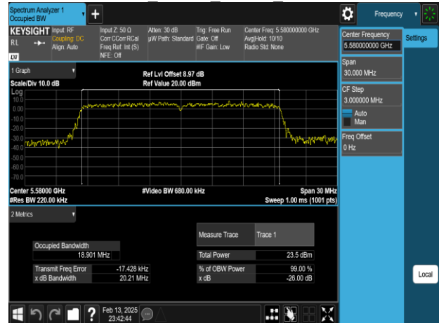
802.11ax 20MHz Chain0 5580MHz
