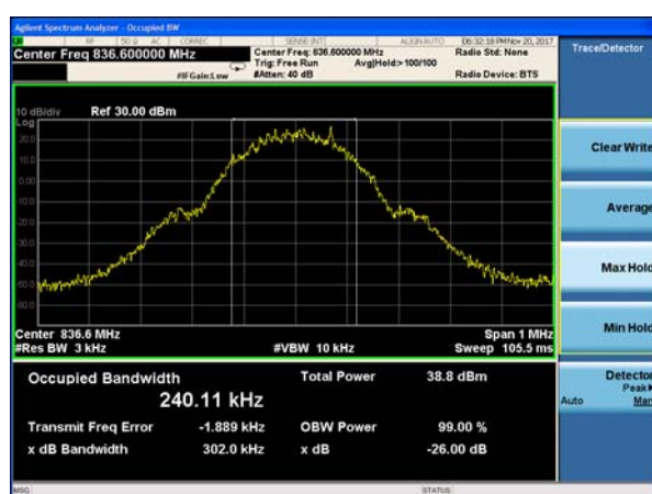
GSM 850 CH-Middle
