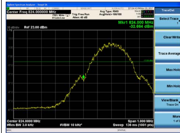
GSM 850 CH-Low
