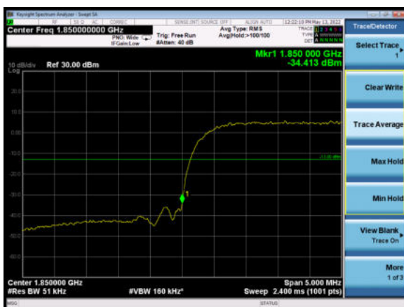
LTE Band 2 1.4MHz QPSK 1RB CH-Low
