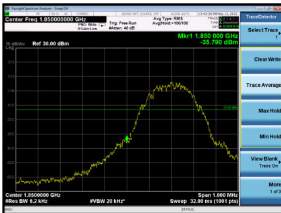
GSM1900 EGPRS CH-Low
