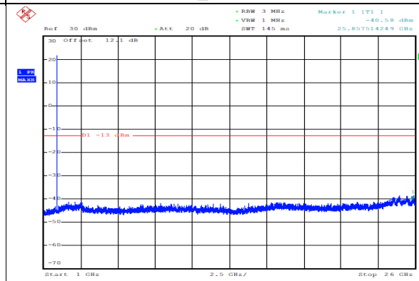
GSM1900_EDGE_661_1000MHz-26000MHz _CSE
