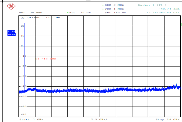
GSM1900_EDGE_810_1000MHz-26000MHz _CSE
