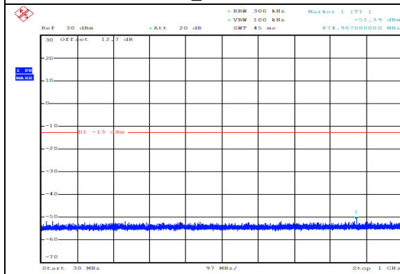
GSM1900_EDGE_810_30MHz-1000MHz _CSE
