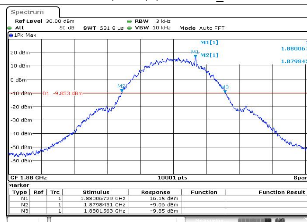
GSM1900,GSM,0,1880MHz_OBW
