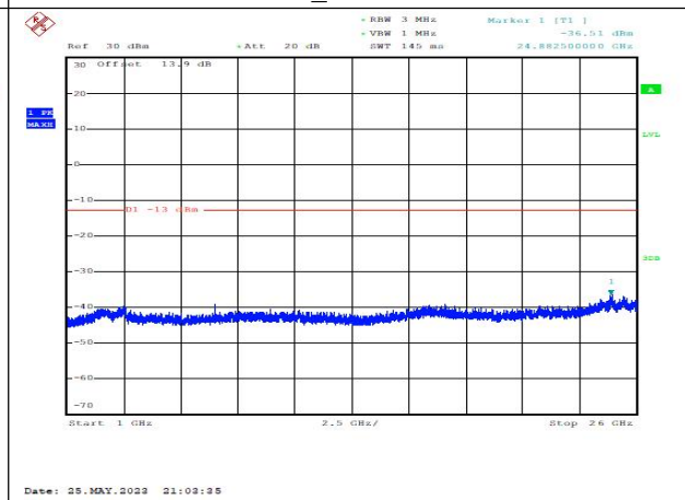
GSM850_EDGE_251_1000MHz-26000MHz_CSE
