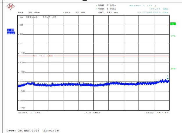
GSM850_GPRS_251_1000MHz-26000MHz_CSE
