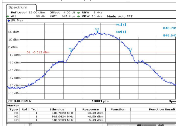
GSM850,EDGE,6,848.8MHz_OBW
