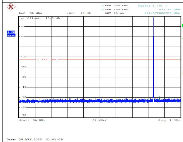
GSM850_GPRS_251_30MHz-1000MHz_CSE
