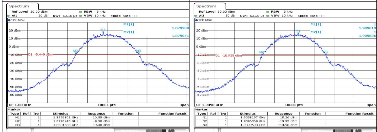
GSM1900,GPRS,3,1880MHz_OBW
