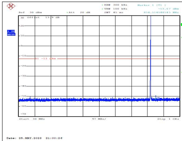
GSM850_GPRS_189_30MHz-1000MHz_CSE
