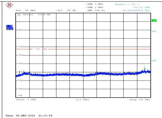
GSM850_GPRS_189_1000MHz-26000MHz_CSE
