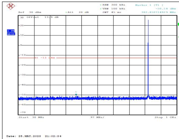
GSM850_EDGE_189_30MHz-1000MHz_CSE
