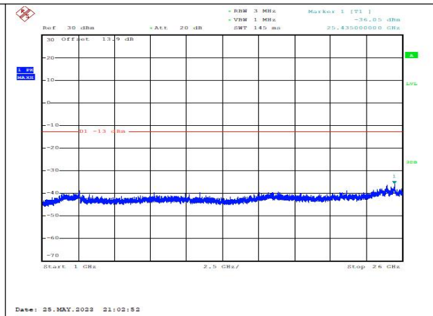
GSM850_EDGE_189_1000MHz-26000MHz_CSE
