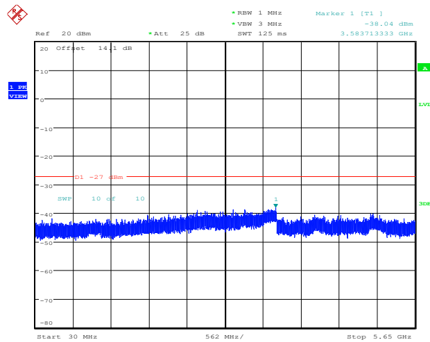
11A_Ant1_5825_30~5650
