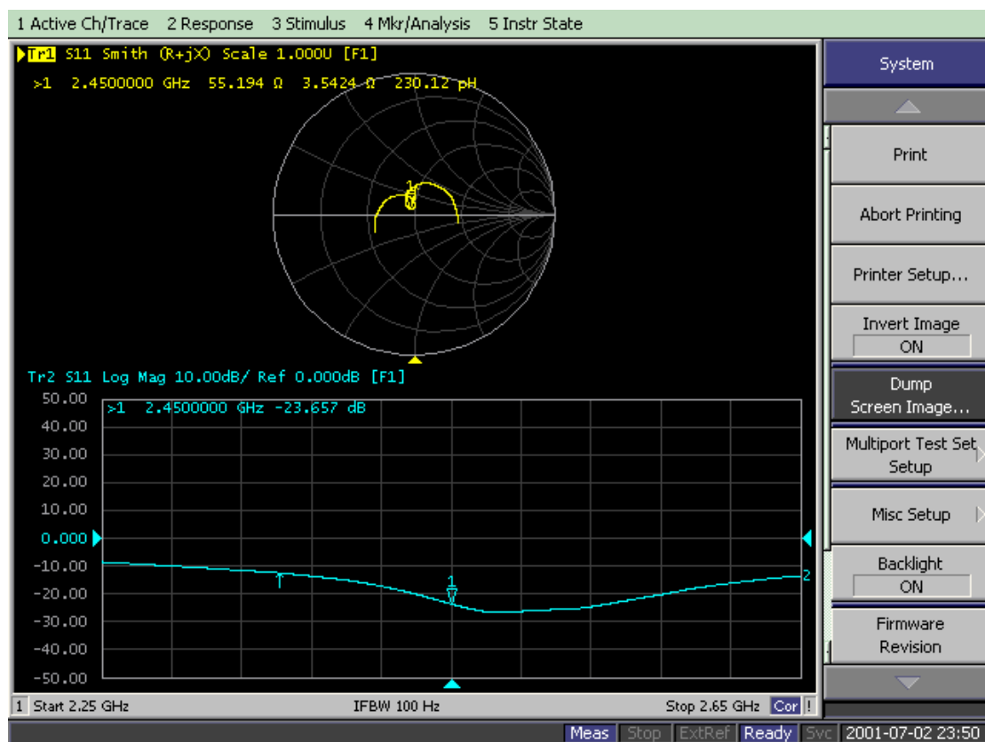
D2450V2-Body-8/28/2018
