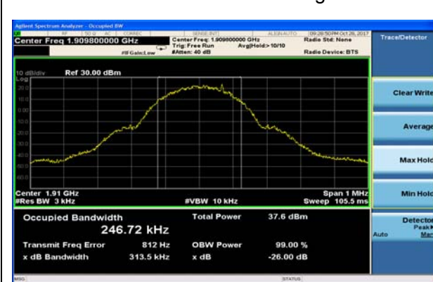
GSM 1900 GSM CH-High
