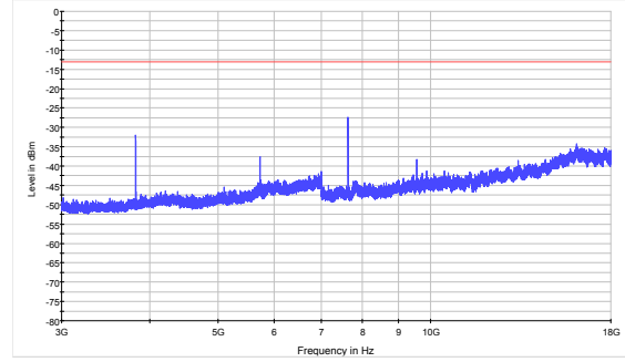
GSM 1900 CH-High 3GHz~18GHz
