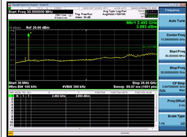
GFSK-CH78
