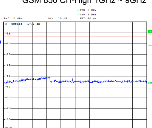
GSM 850 CH-High 1GHz ~ 9GHz
