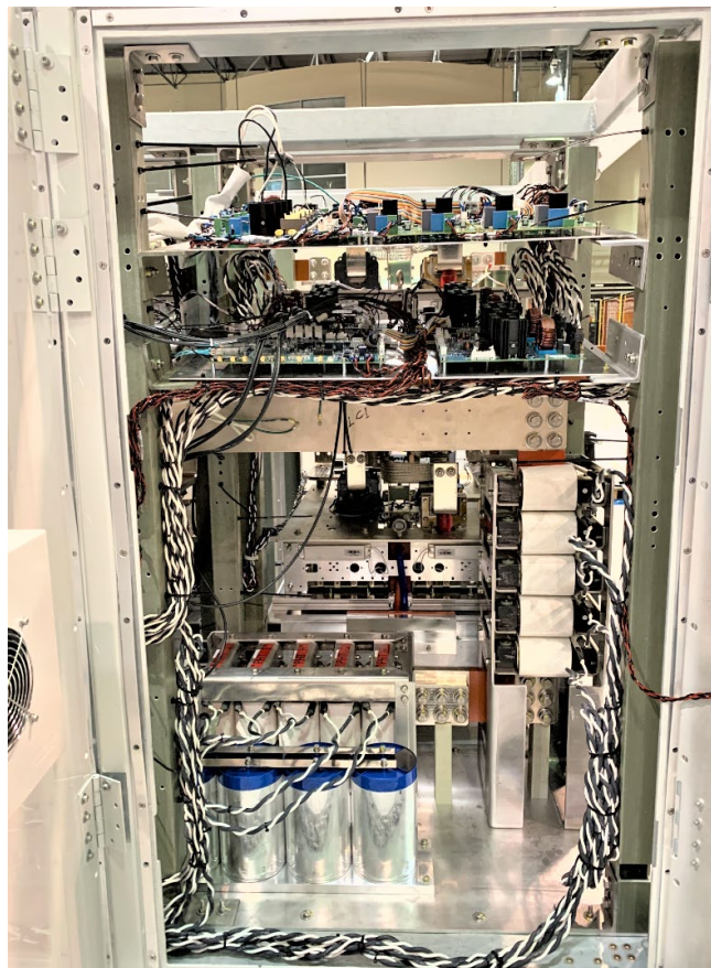
2 MVar. Module
