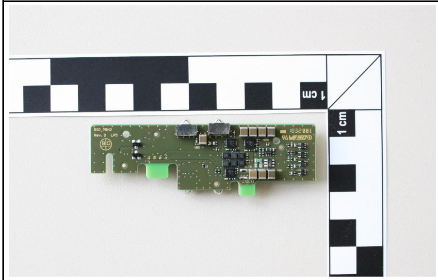
PGH-PCB-LP5-bottom
