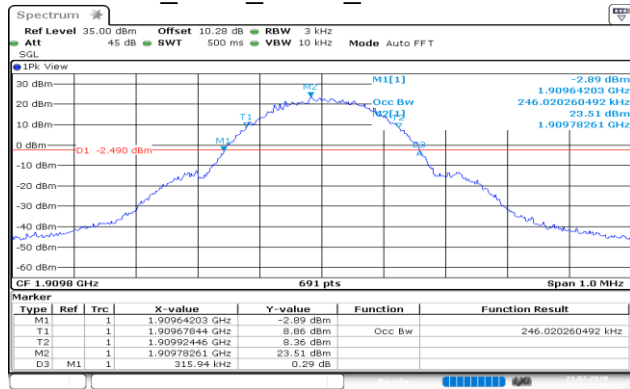
GPRS_1900_Higher_26BW and 99%
