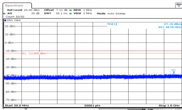
EGPRS_1900(8PSK)_Higher(30MHz-1GHz)
