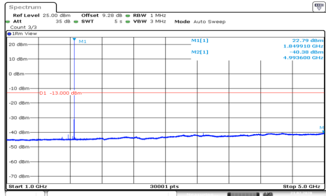
EGPRS_1900(8PSK)_Lower(1GHz-5GHz)
