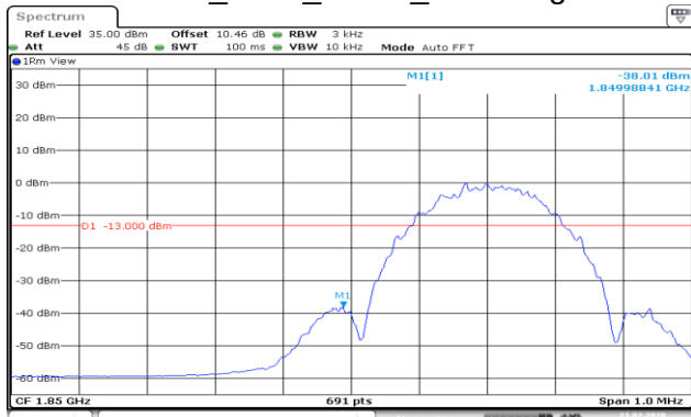
GPRS_1900_Lower_Band edge
