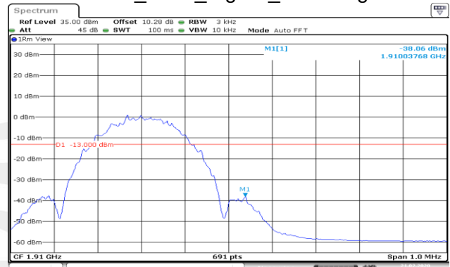
GPRS_1900_Higher_Band edge
