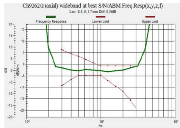
Fig. 7.10 WCDMA Band II Ch9262
