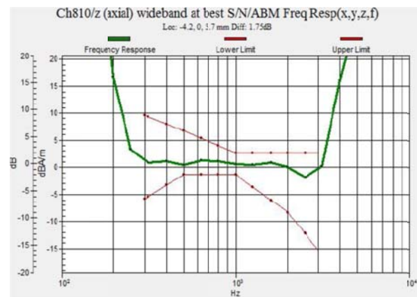
Fig 7.6 GSM1900 Ch810
