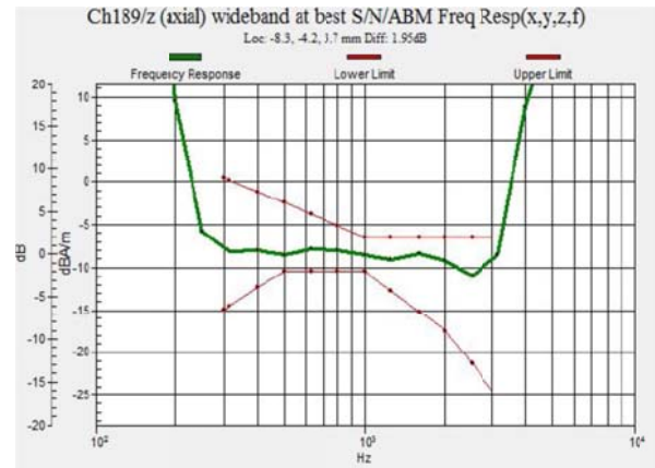
Fig 7.2 GSM850 Ch189
