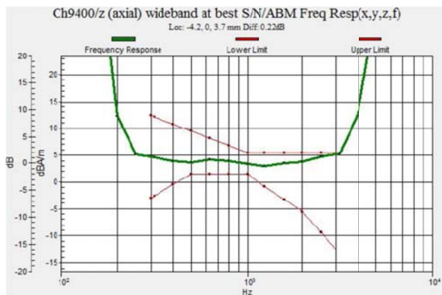
Fig. 8.13 WCDMA Band II Ch9400
