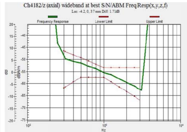
Fig. 7.8 WCDMA Band V Ch4182
