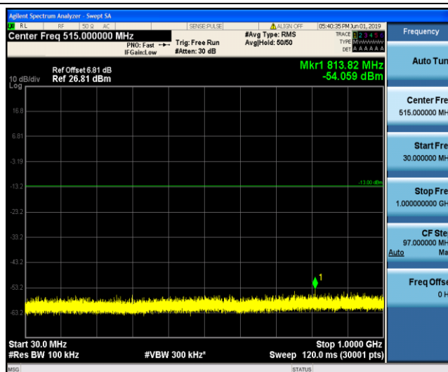
Band2 20MHz 16QAM 18700 1RB#0
